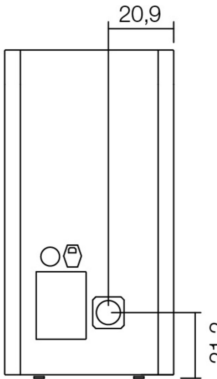
vista retro stufa
